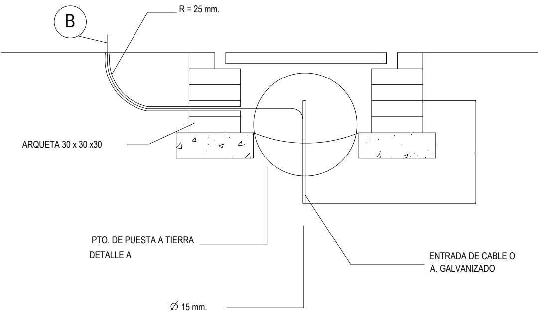
DETALLE A
