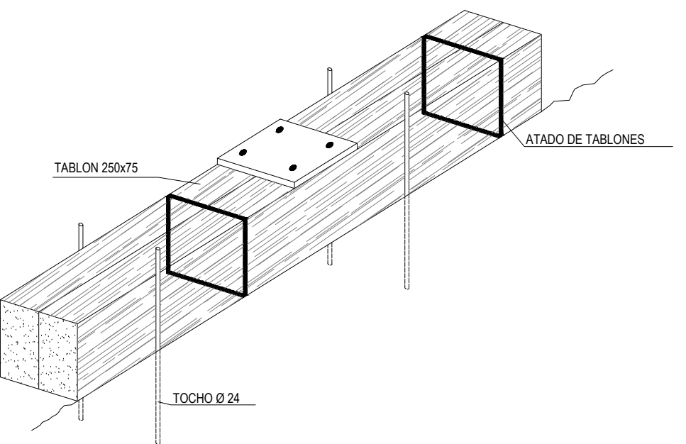
CONJUNTO
