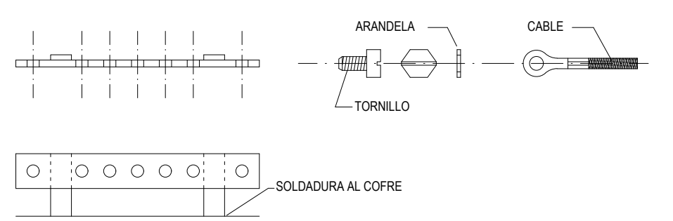
DETALLE DE REGLETA
