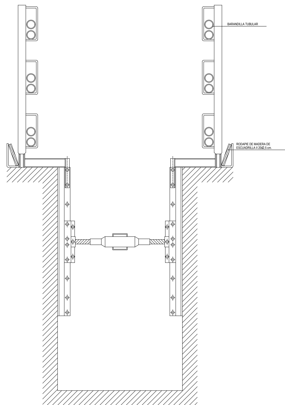
PROTECCION LATERAL
