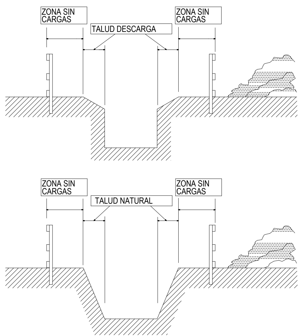
ESQUEMAS DE PROTECCIONES DE ZANJAS
