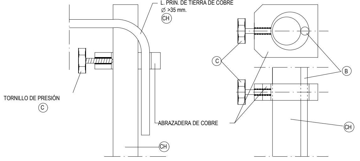
DETALLE A
