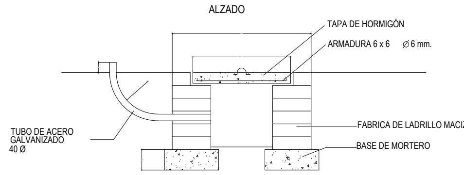
DETALLE DE ARQUETA
