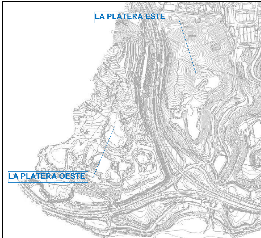
Figura Nº 1.- Plano topográfico de la finca de La Platera (FYM, 2017).
