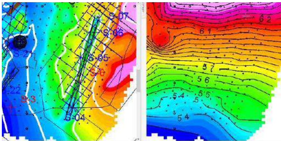
Figura Nº 16.- Anomalía de Bouguer 2.67g/cm 3 comparada con el grid de elevaciones..
