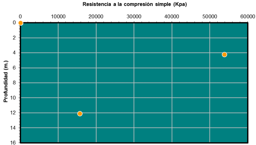
Figura Nº 96.- Valores de compresión simple en relación a la profundidad.
