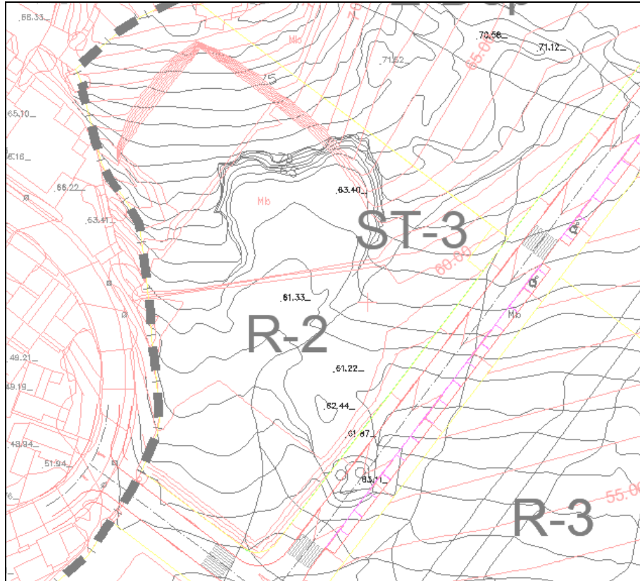
Figura Nº 123.- Modificación topográfica propuesta para la parcela R-2.
