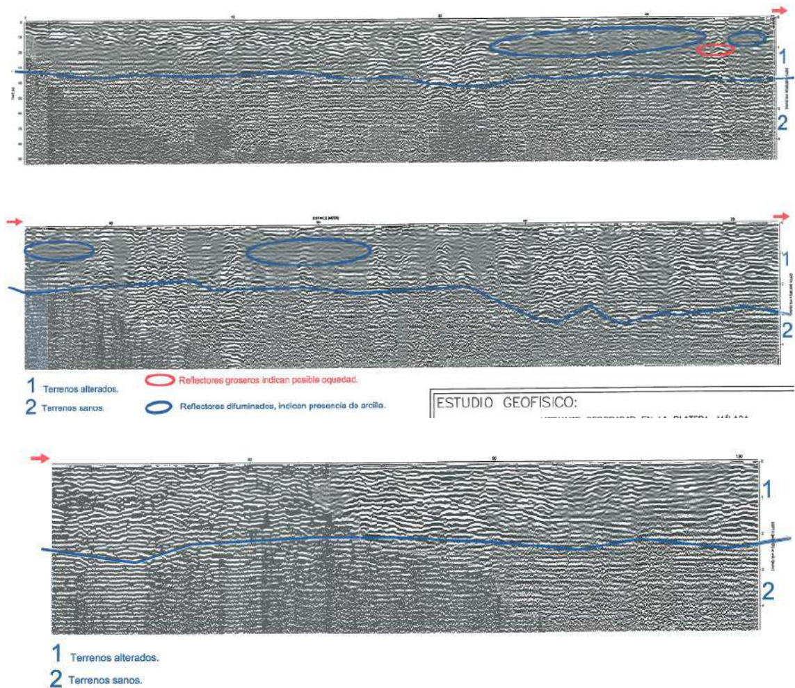
Figura Nº 36.- Interpretación del perfil GPR-15.
