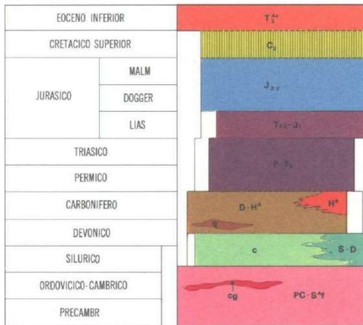
Figura Nº 8.- Reproducción de mapa geológico MAGNA, Hoja de Málaga 1053/17-44
