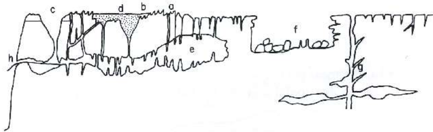
Figura Nº 103.- Morfología de un macizo calcáreo. a) Lapiaz desnudo. b) Lapiaz cubierto. c) Dolina. d) Dolina cubierta. e) Cueva. f) Torca. g) Sima. h) Fuente.
