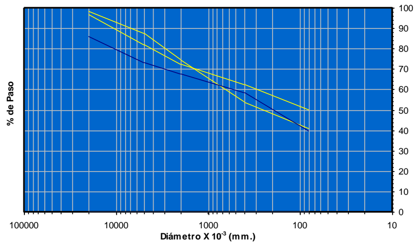
Figura Nº 57.- Distribución de curvas granulométricas.
