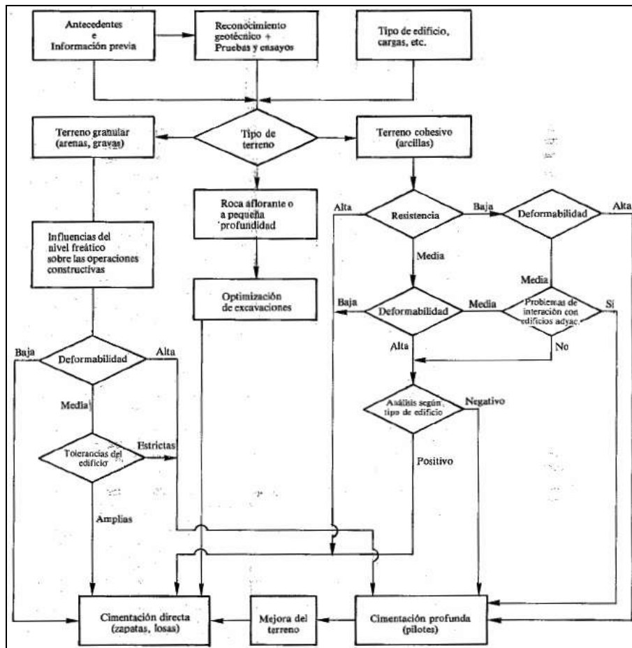
Figura Nº 131.- Esquema de decisión en la selección de cimentación (Rodríguez Ortiz, 1972).
