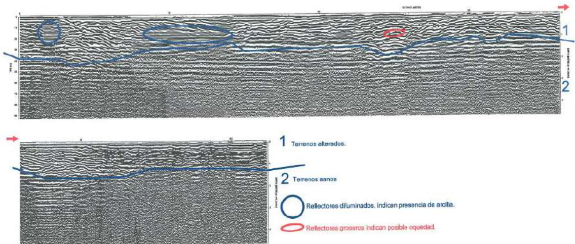
Figura N° 22.- Interpretación del perfil GPR-01.
