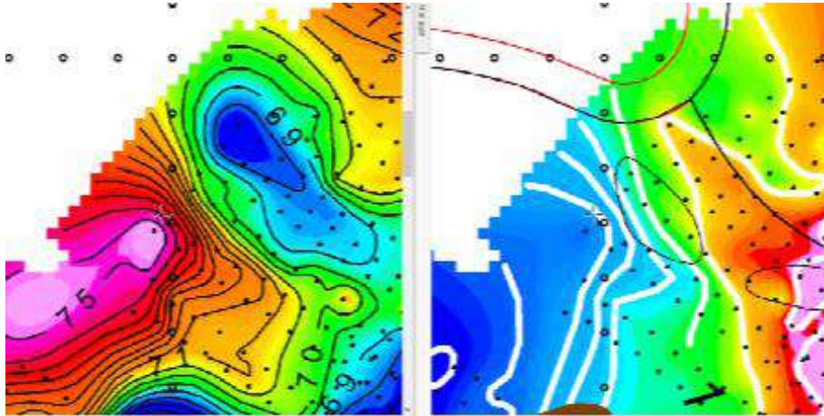
Figura Nº 15.- Anomalía de Bouguer 2.67g/cm 3 comparada con el grid de elevaciones..
