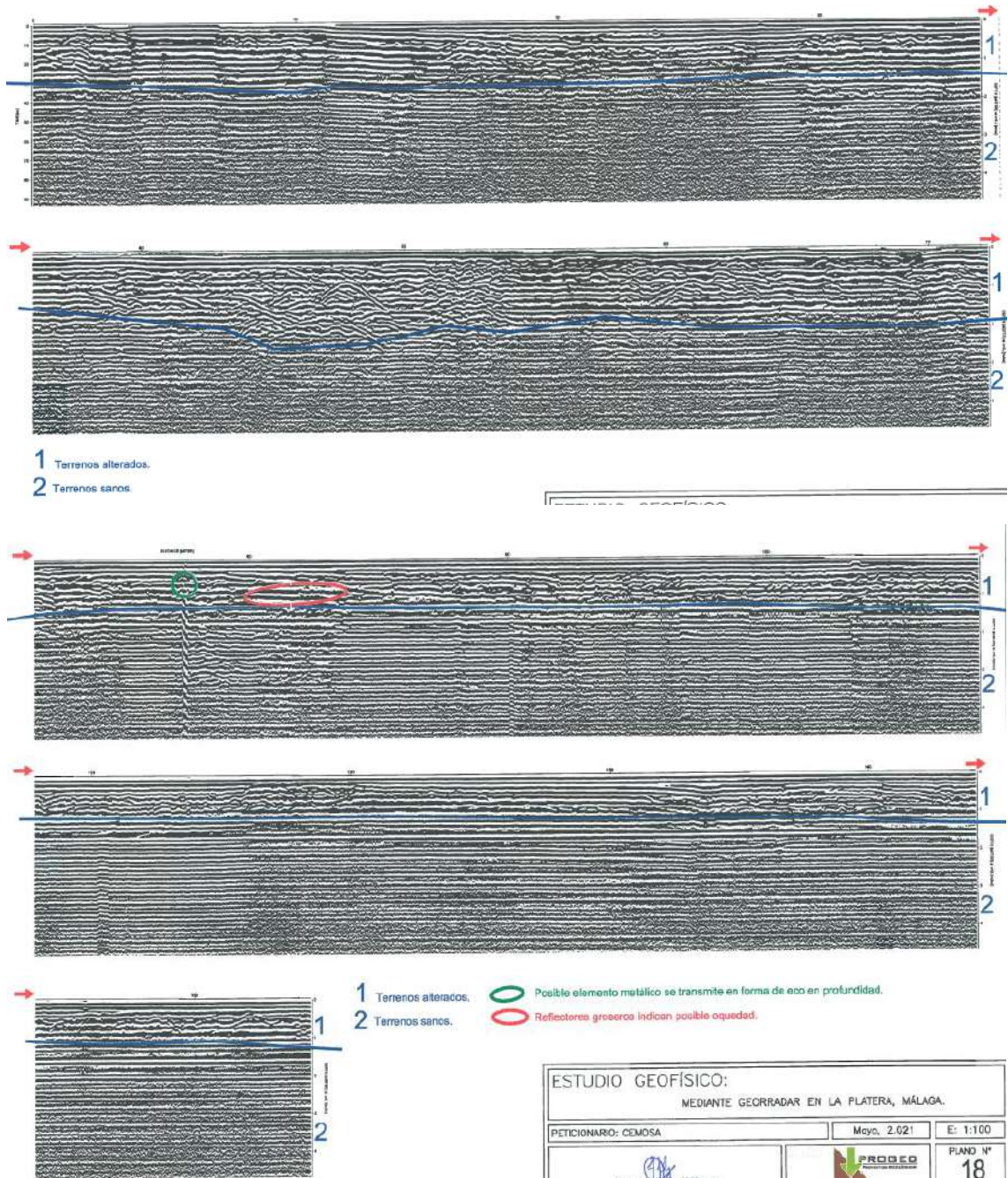
Figura Nº 35.- Interpretación del perfil GPR-14.
