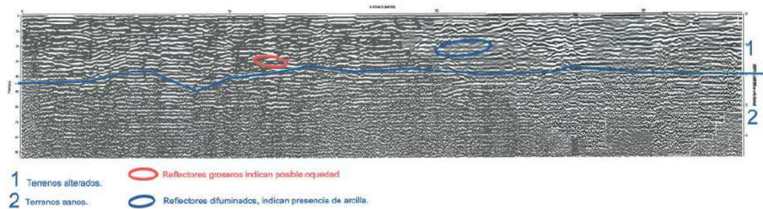
Figura Nº 40.- Interpretación del perfil GPR-19.
