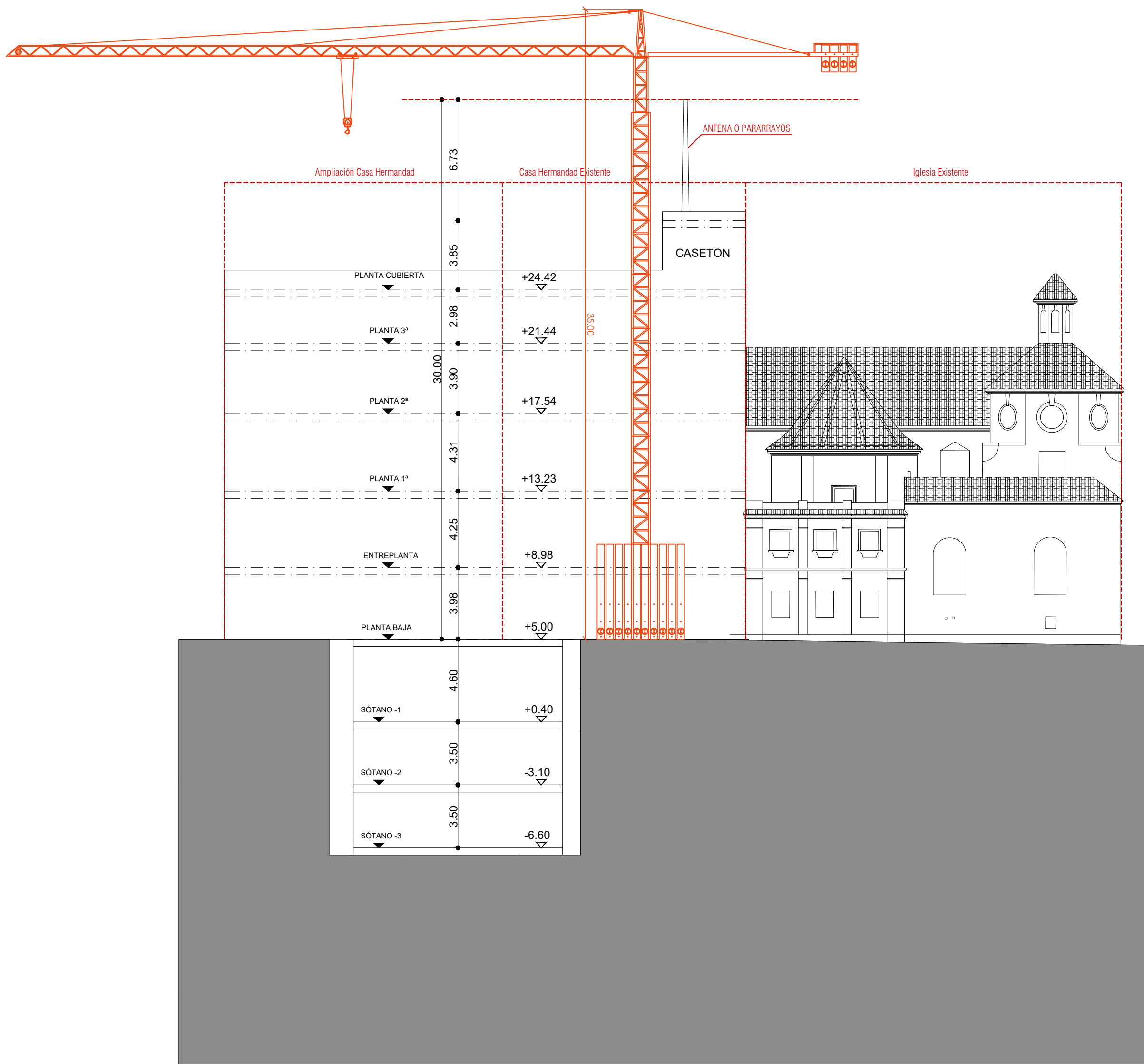
SECCIÓN A-A
