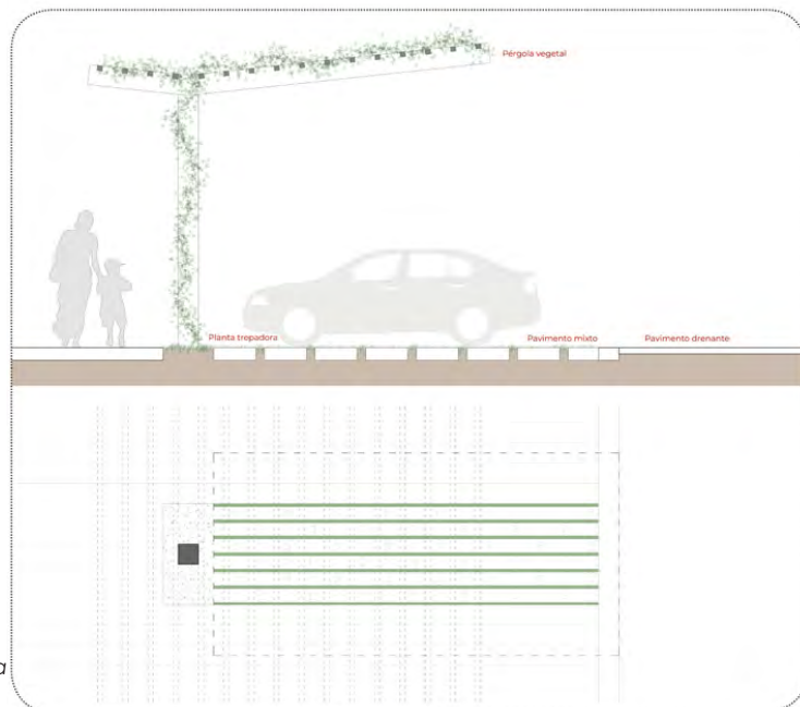
Sección propuesta para mejora de viario y aparcamientos
