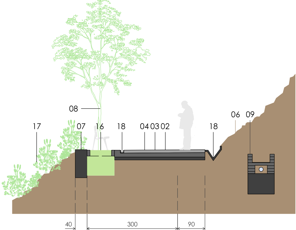
Sección C: Camino en zonas con terraplén sin acueducto visible
