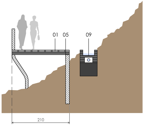
Sección A: Caminos en zonas escarpadas
