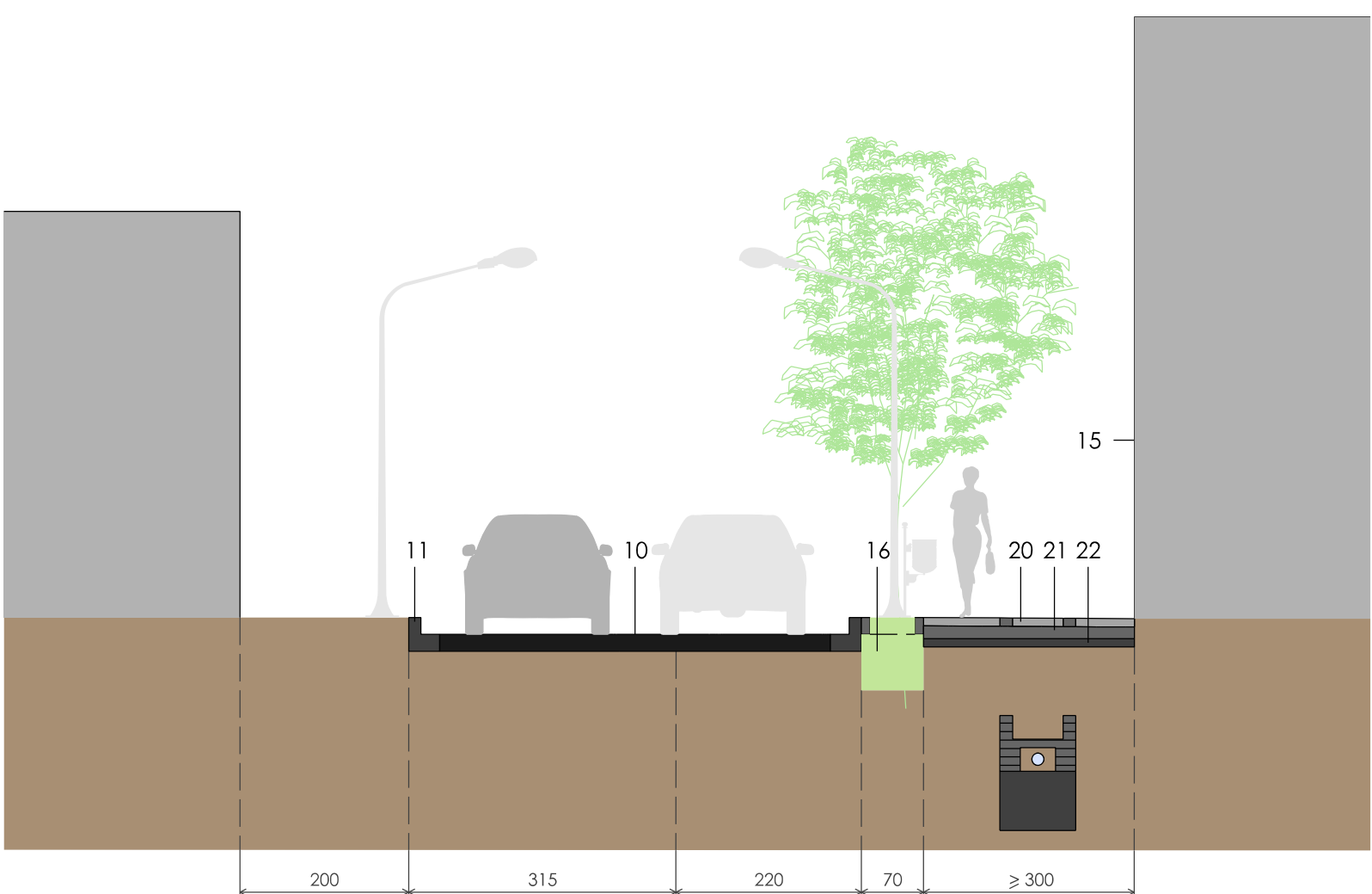
Sección F: Centro de ciudad
