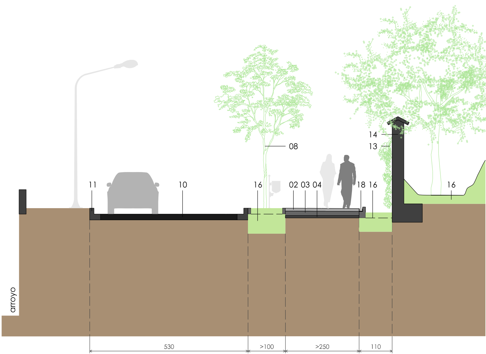
Sección E: Camino en zonas urbanas con edificaciones (UA-V5) (UA-V12)
