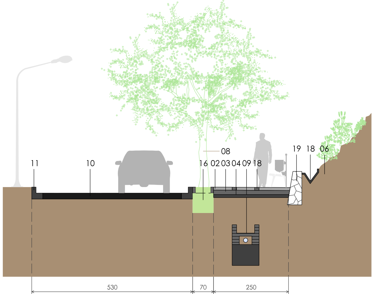
Sección D: Zonas urbanas con taludes naturales
