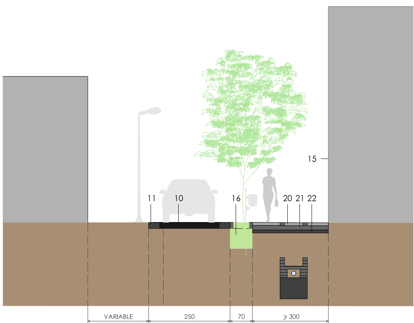
Sección G: Tramo de preferencia peatonal
